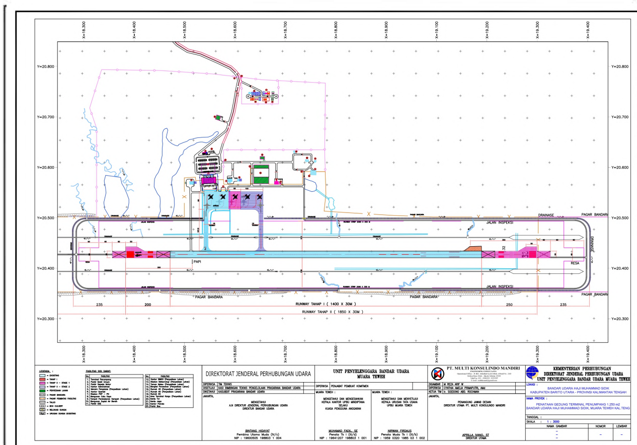
Gambar 1. 1 Layout Bandar Udara Haji Muhammad Sidik
